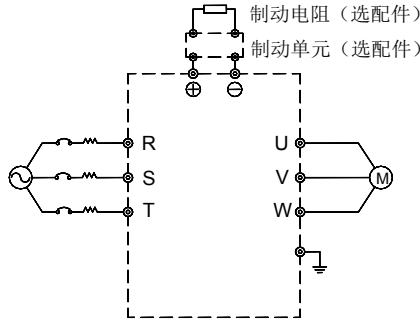
图 3-3 主回路标准接线
