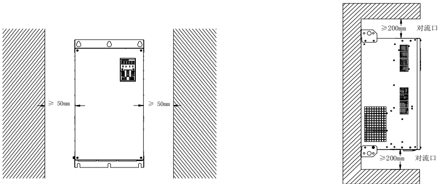
图 2-2 变频器安装方向和空间
