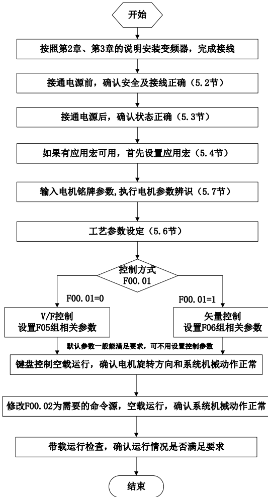
图 5-1 变频器调试流程图
